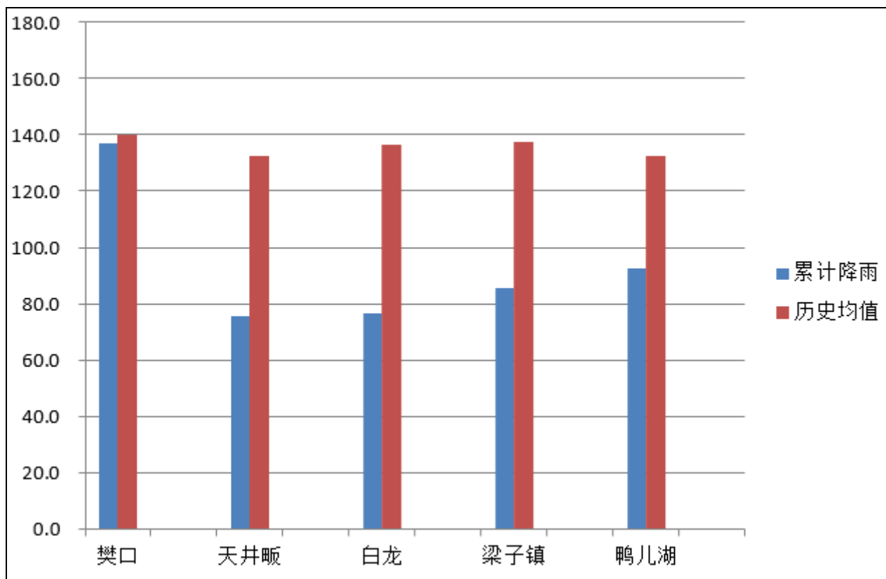
图 1 鄂州市 4 月降雨总量比较图（单位：mm）
