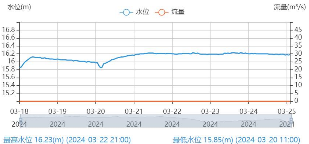
图 2 樊口大闸上（内港）一周以来水位变化图
