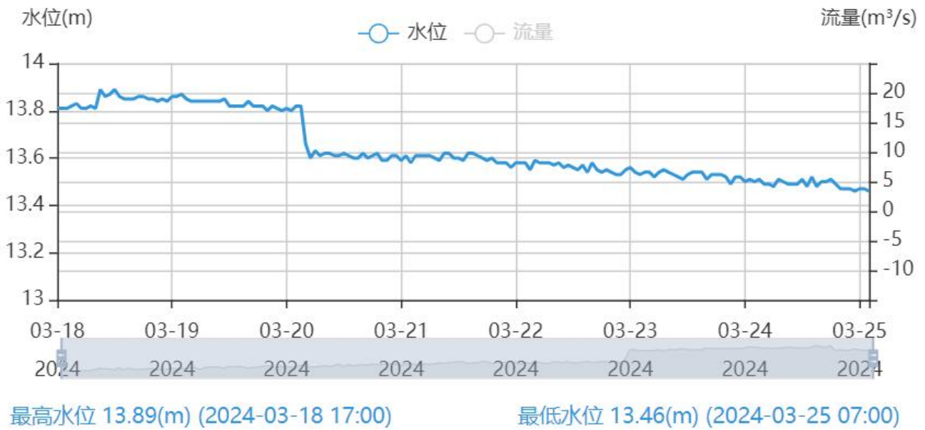
图 1 长江鄂州段一周以来水位变化图
